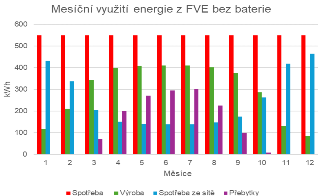
Obr. 27 Měsíční využití energie z FVE bez baterie
