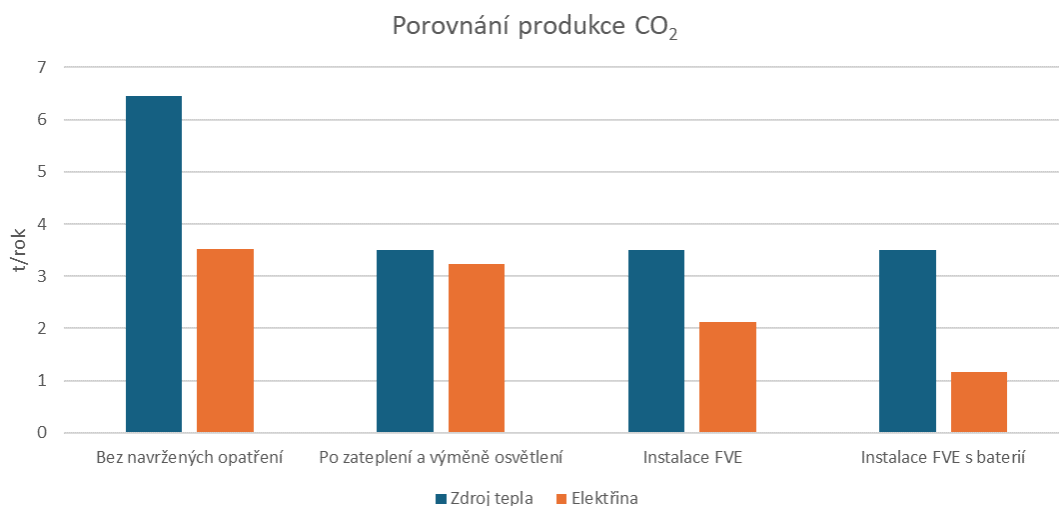
Obr. 31 Uhlíkové stopa návrhových opatření
