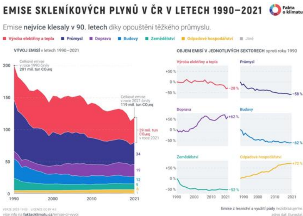
Obr. 41 Vývoj skleníkových plynů v ČR (zdroj: Fakta o klimatu)
