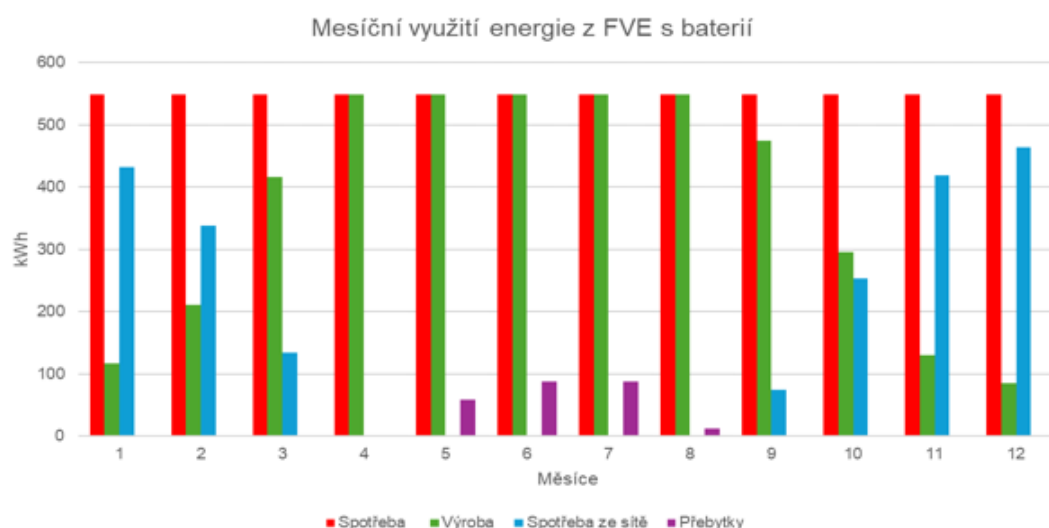
Obr. 30 Měsíční využití energie z FVE s baterií
