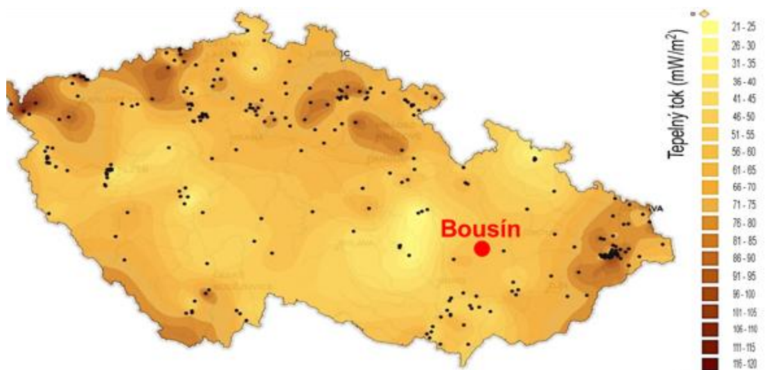
Obr. 13 Geotermální potenciál ČR (zdroj: Česká geologická služba)
