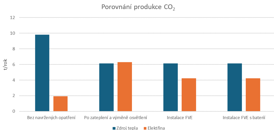
Obr. 28 Uhlíková stopa návrhových opatření
