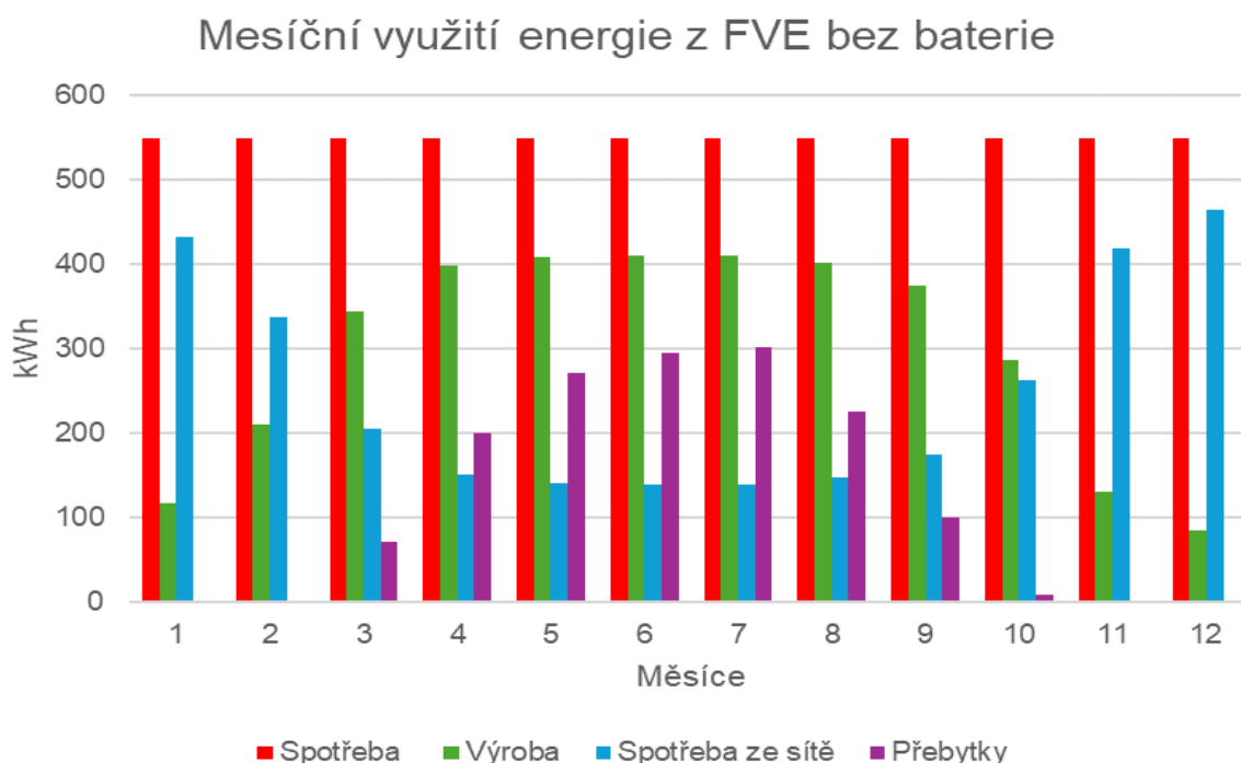
Obr. 27 Měsíční využití energie z FVE bez baterie
