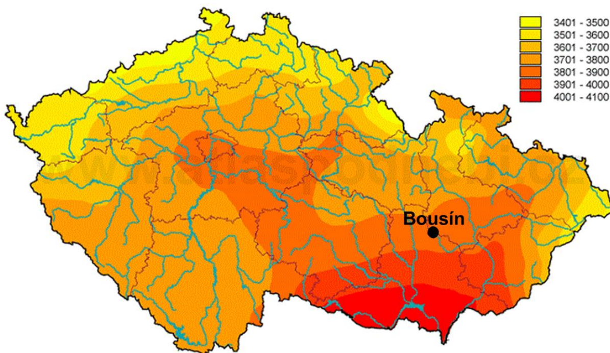
Obr. 16 Roční dávky slunečního záření na vodorovnou plochu v ČR (MJ/m 2 ·rok -1 ) (zdroj: ČHMÚ)
