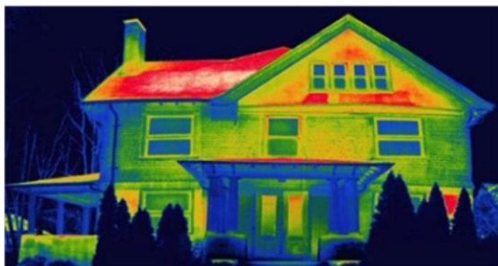
Obr. 36 Termovizní měření tepelných ztrát (zdroj: Getty Images)
