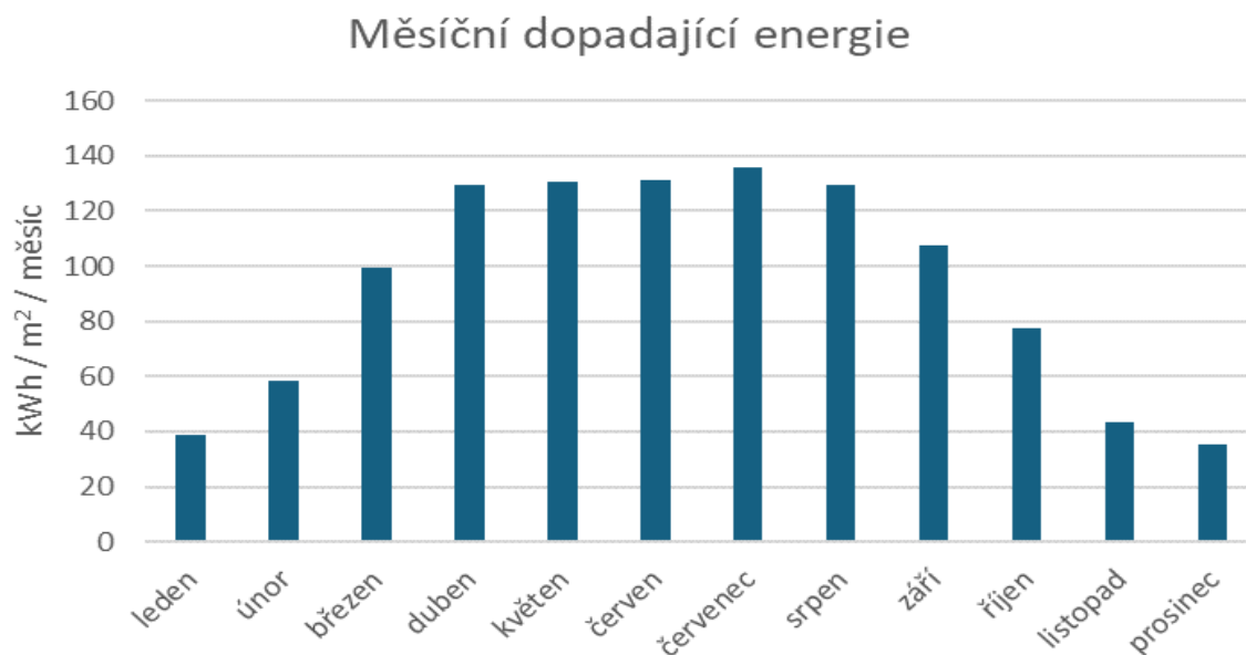
Obr. 18 Sluneční energie při optimálních podmínkách na m² v různých měsících (zdroj: PVGIS)
