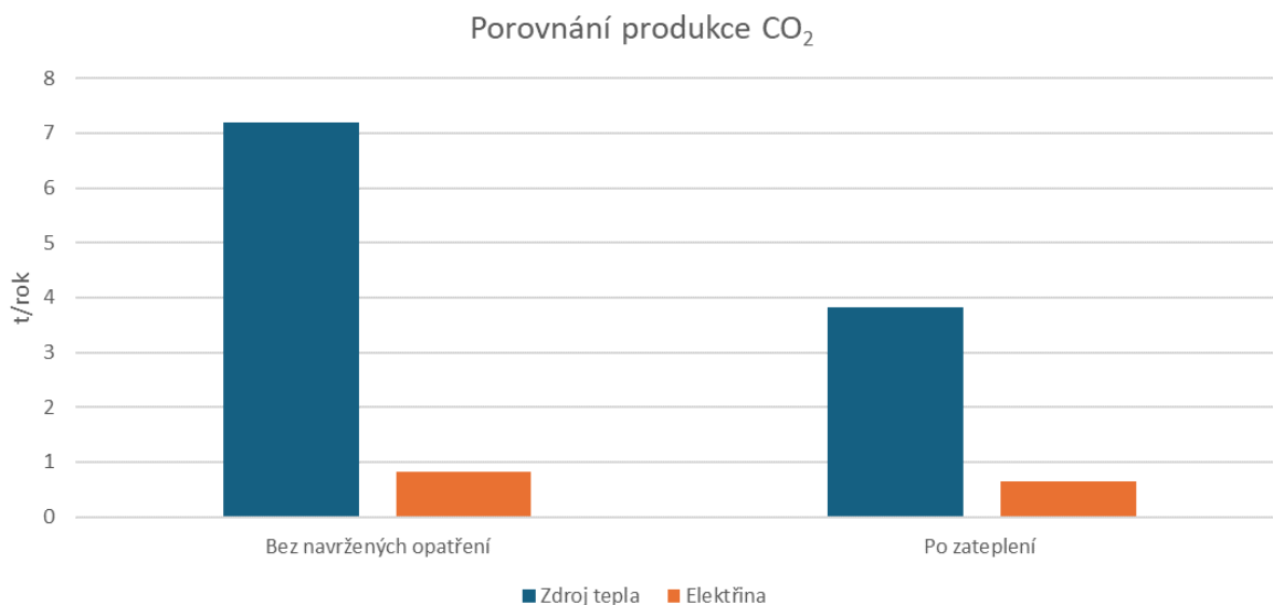
Obr. 32 Uhlíková stopa návrhových opatření
