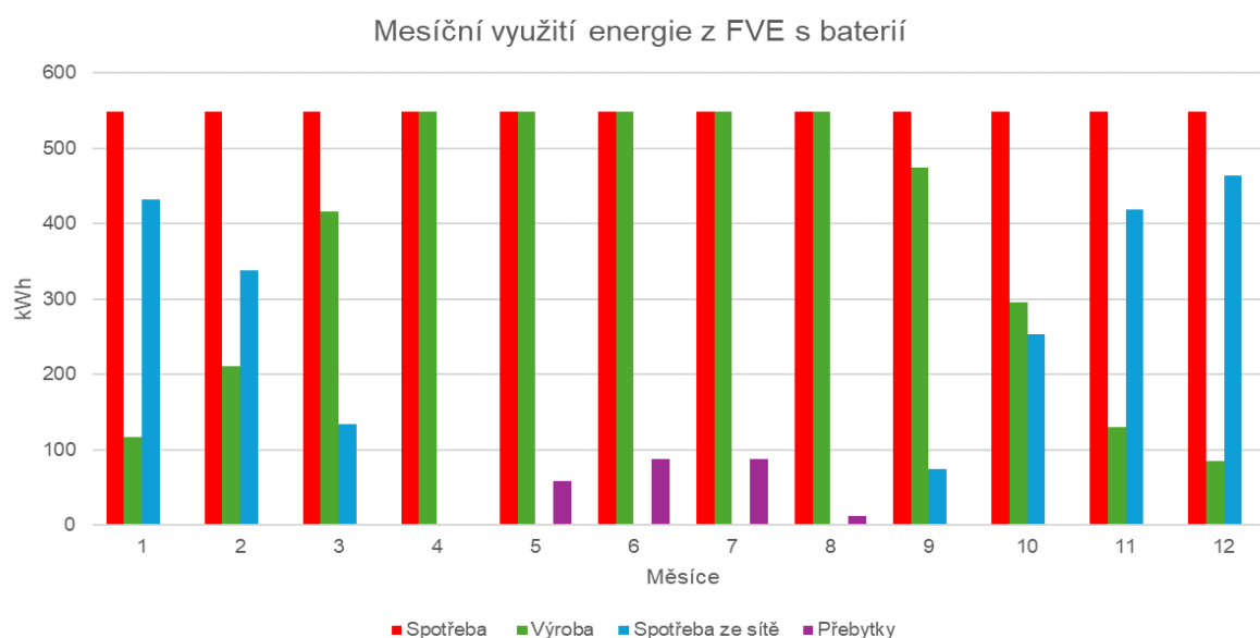
Obr. 30 Měsíční využití energie z FVE s baterií
