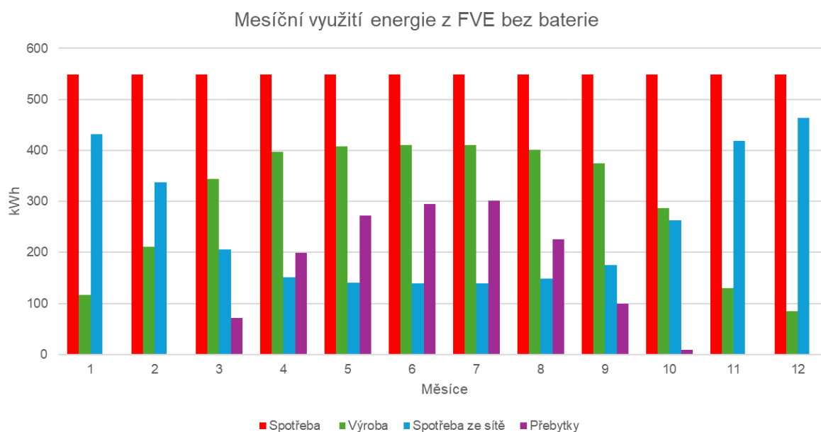
Obr. 29 Měsíční využití energie z FVE bez baterie
